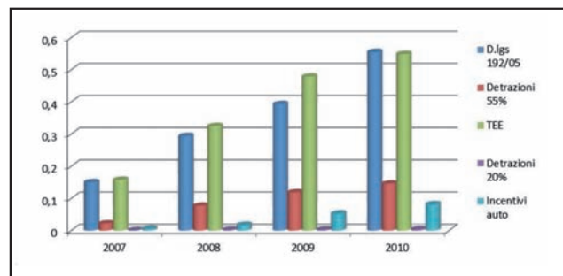
FIGURA 4 Efficacia delle misure espressa in GWh risparmiati
