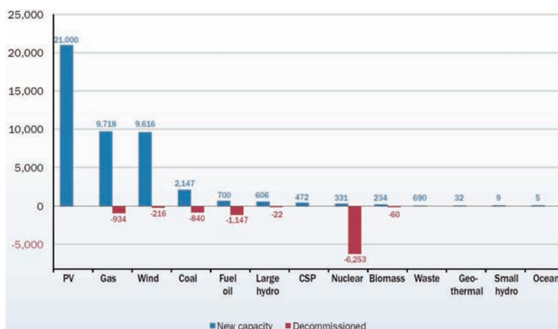
FIGURA 1 Nuova potenza installata e dismessa nel settore elettrico europeo nel 2011 (MW) Fonte: EWEA
