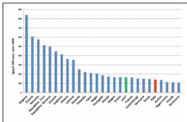
FIGURA 2 Intensità energetica primaria UE27, anno 2009 (ktep/1.000€)
