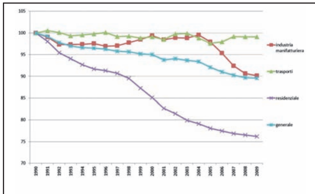
FIGURA 3 Indici di efficienza energetica (1990=100) Fonte: elaborazione ENEA su dati MISE
