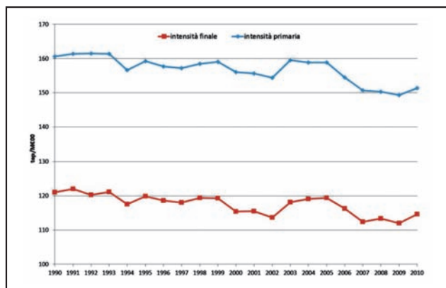
FIGURA 1 Intensità energetica primaria e finale nel periodo 1990-2010 (tep/M€00)
