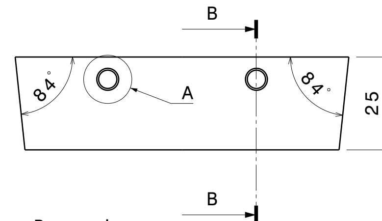
Rear view Scale: 1:1
