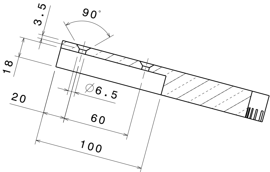
SEZIONE B - B
