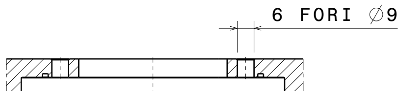
SEZIONE D - D
