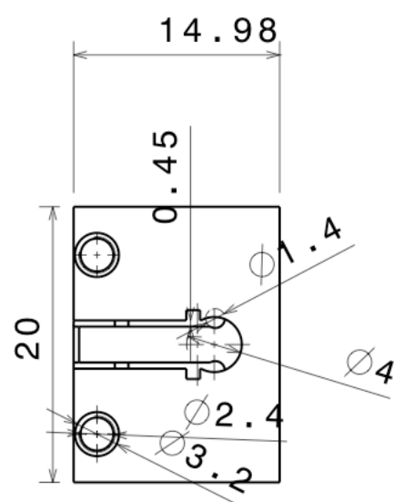
Right view Scale: 2:1
