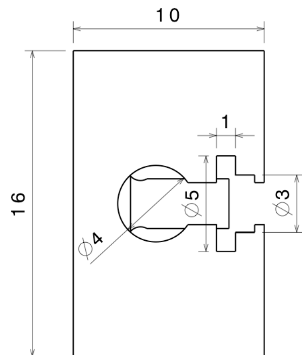
Left view Scale: 5:1
