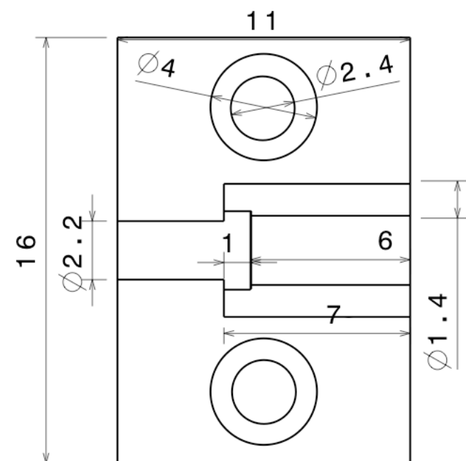
Front view Scale: 5:1
