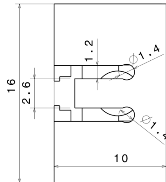
Right view Scale: 5:1
