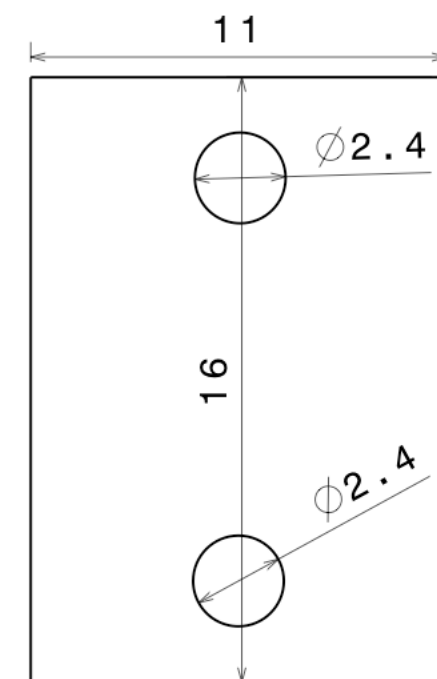
Rear view Scale: 5:1
