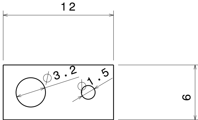
Piastrina Front view Scale: 4:1
