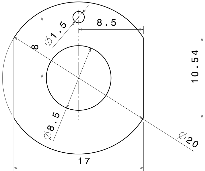
Rondella-A Front view Scale: 4:1
