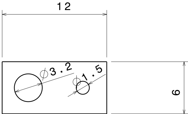
Piastrina-B Front view Scale: 4:1
