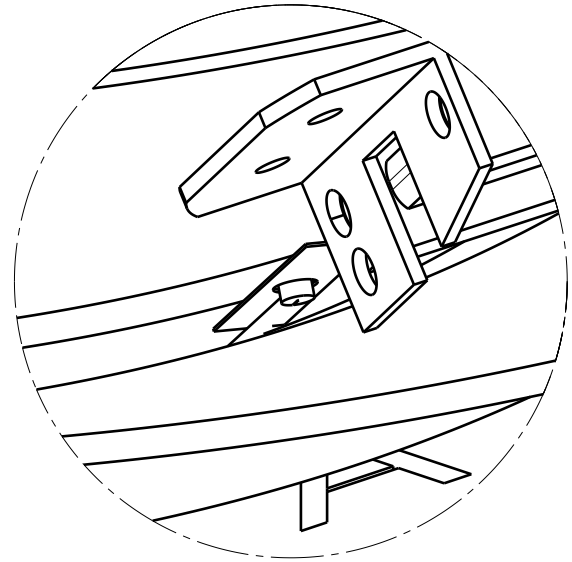
Detail B Termocoppia Schermo Conico Scale: 2:1
